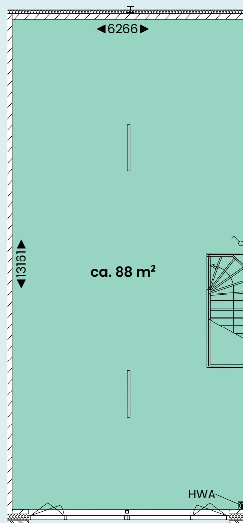
EERSTE VERDIEPING
