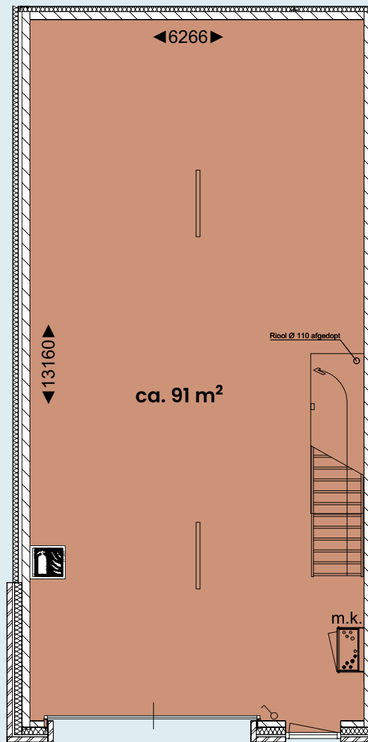
BEGANE GROND
